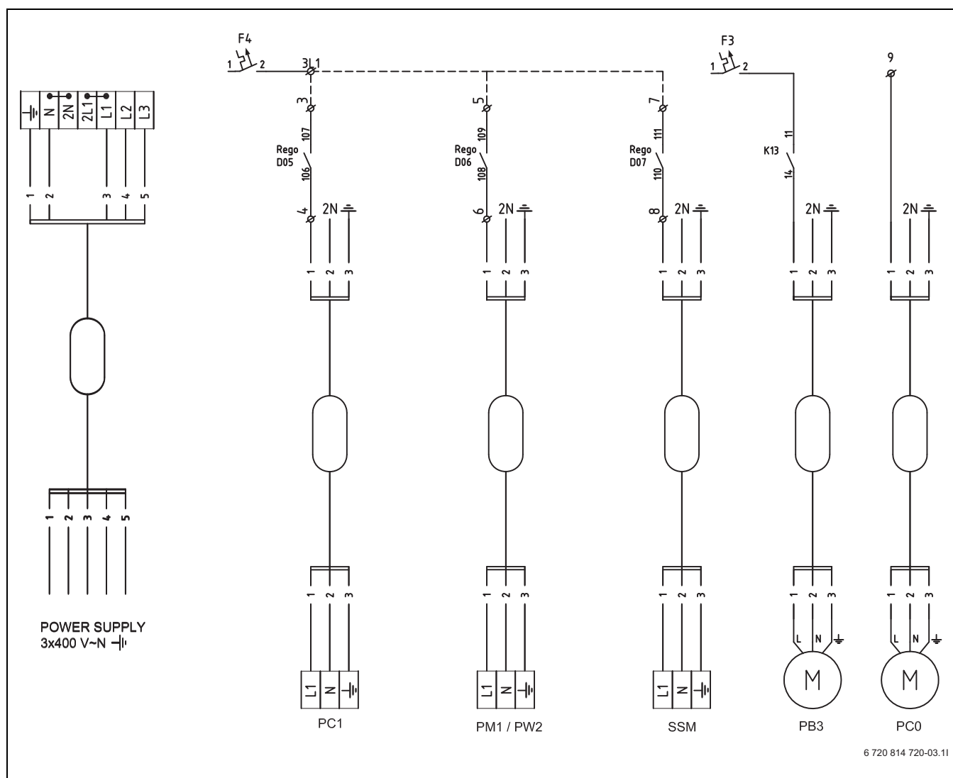
Kuva 15 Ulkoisten liitântöjen kytkentäkaavio, lämpöpumppu 54–80 kW
