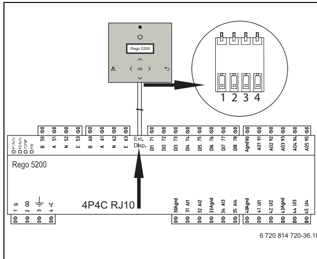
Kuva 12 Rego-näyttö kytkettynä liitännään Ext. Disp Rego-rasiassa
