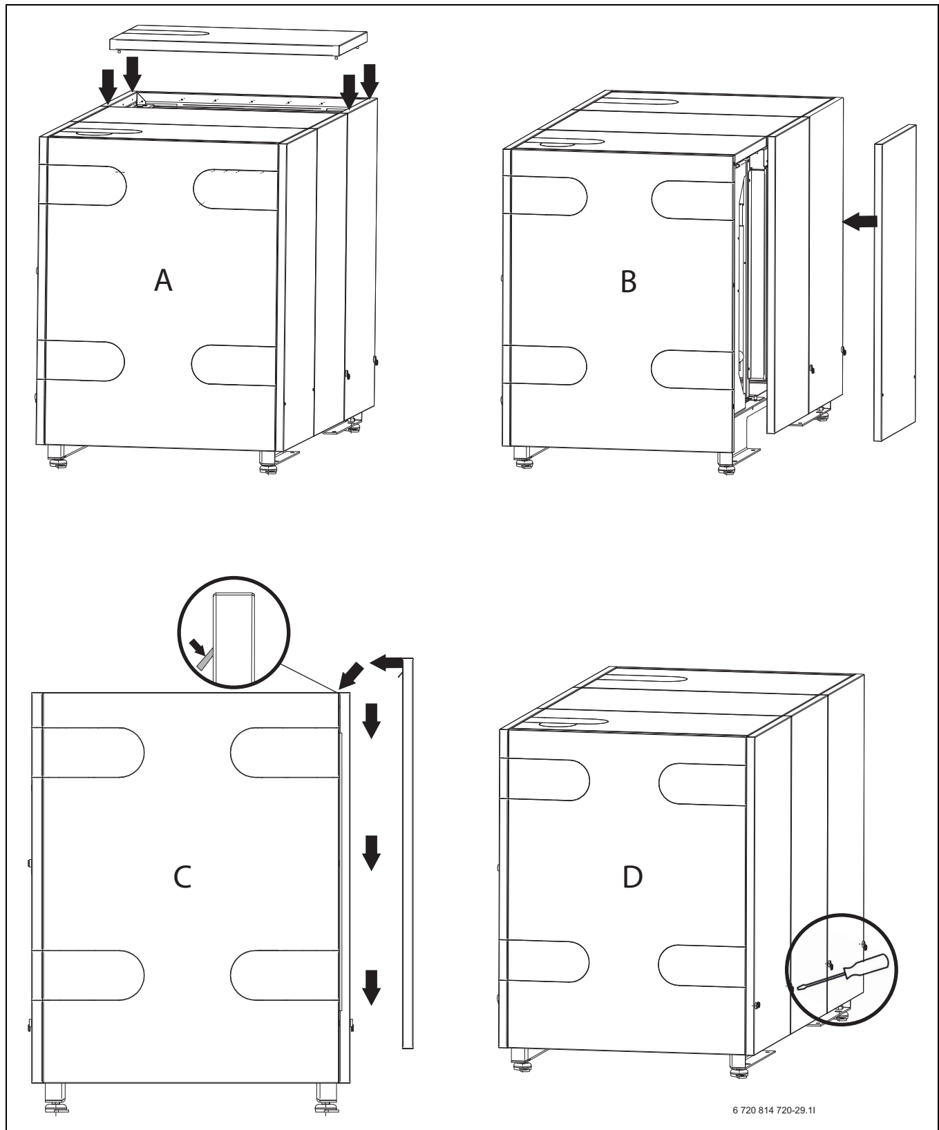
Kuva 8 Suojapeltien asentaminen/irrottaminen
