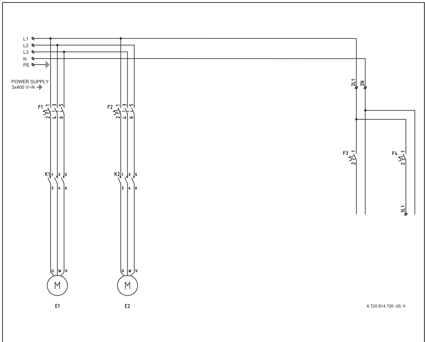
Kuva 17 Pääsyötön piirikaavio, lämpöpumppu 54–80 kW, koskettimella (K1/K2)
