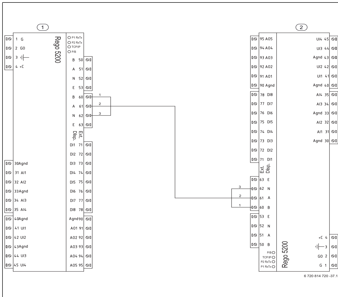
Kuva 21 Kaskadikytcentä 54–80 kW
