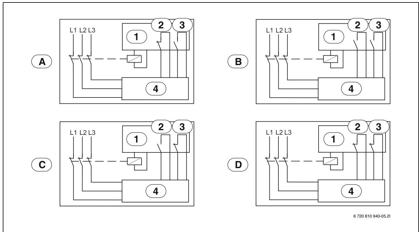
Kuva 25 Kytchentäkaavio EVU/SG
