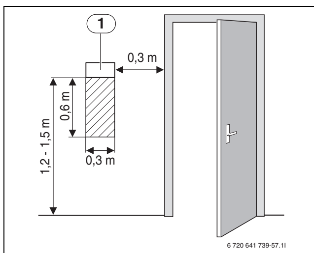
Kuva 10 Suositeltu asennuspaikka huoneanturille
