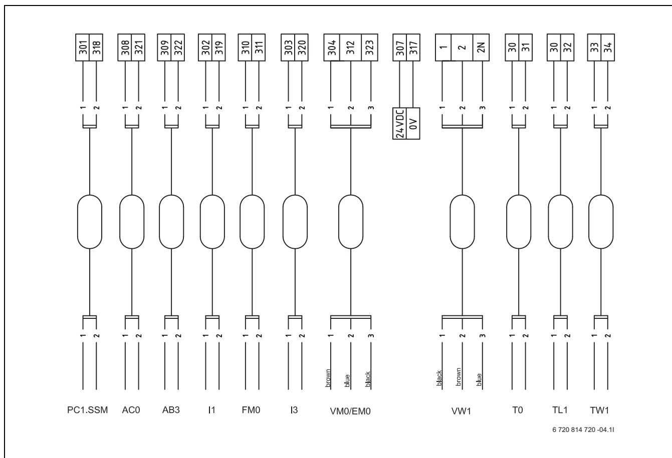
Kuva 16 Ulkoisten liitântöjen kytkentäkaavio, lämpöpumppu 54–80 kW
