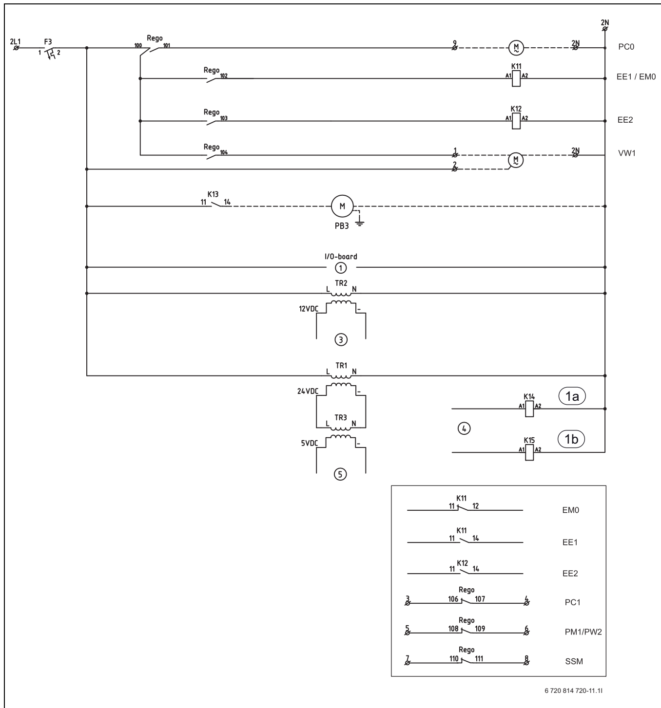
Kuva 24 Piirikaavio 54–80 kW
