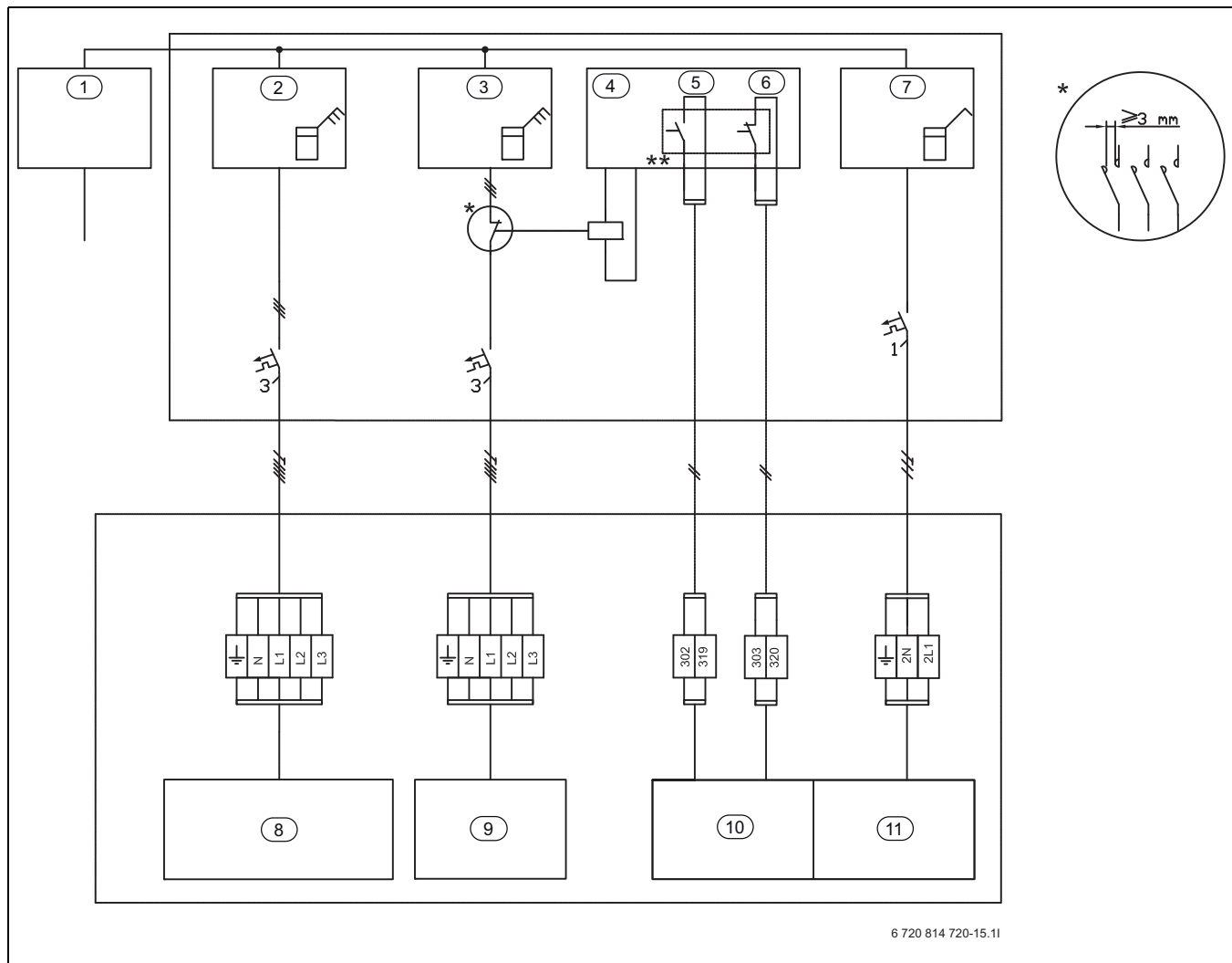
Kuva 26 EVU, tyyppi 1
